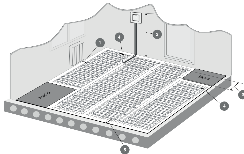
Рис. 1 Приклад укладки нагрівального мату
